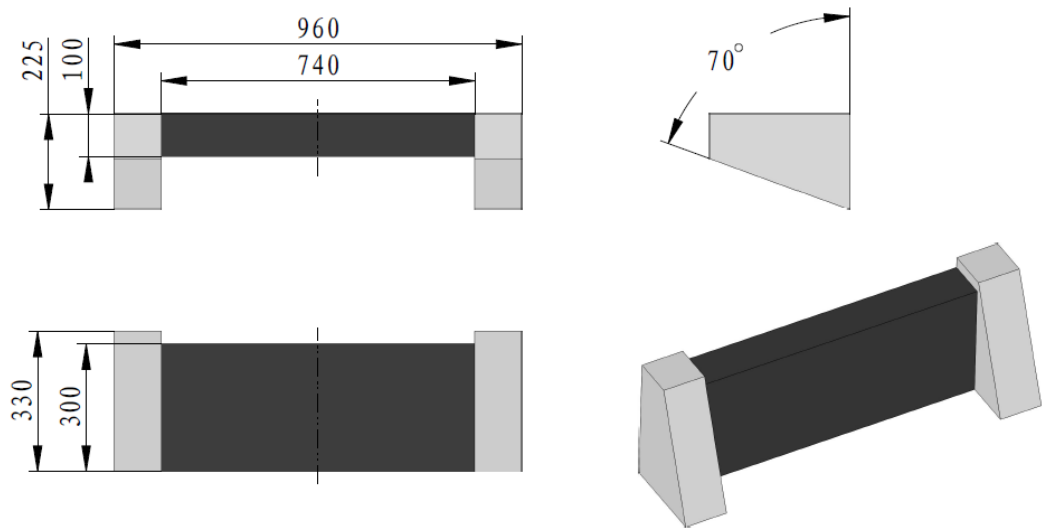
图 二-22 高墙示意图
