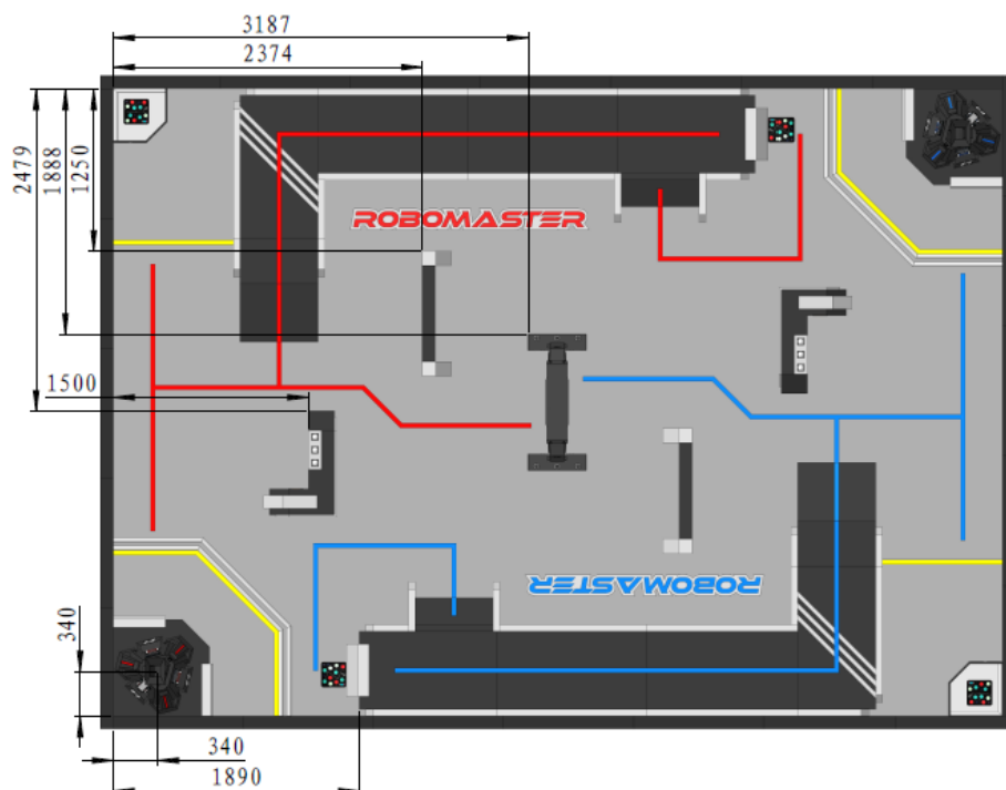
图 二-5 战场模块定位尺寸图
