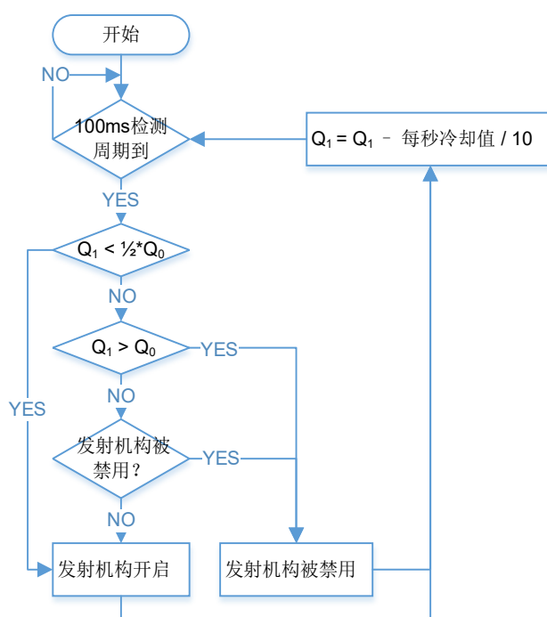
图 三-9 枪口热量冷却逻辑
