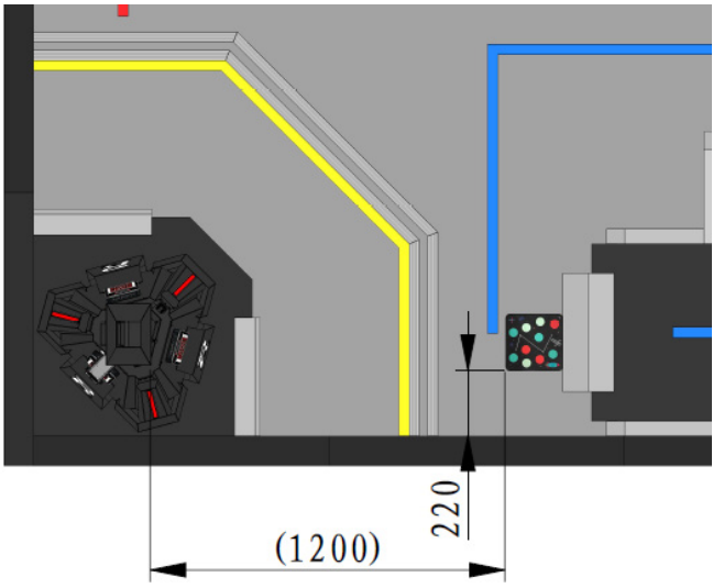
图 二-20 空中机器人识别卡
