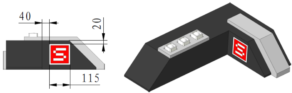
图 二-21 防御标签示意图
