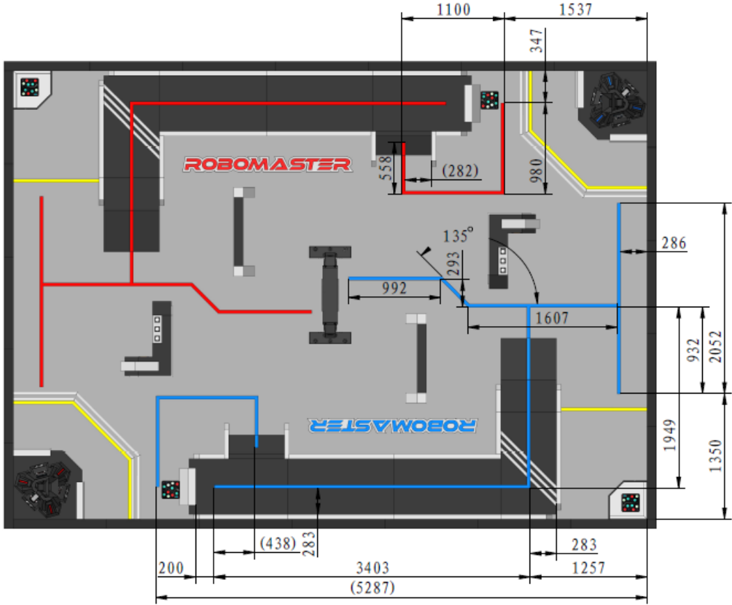
图 三-3 场地引导线
