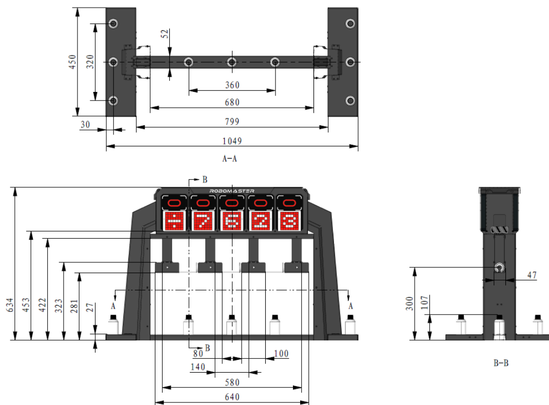
图 二-24 资源岛尺寸图
