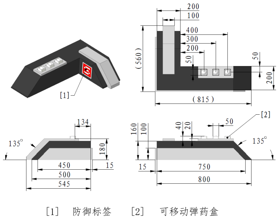
图 二-19 L 地形块示意图
