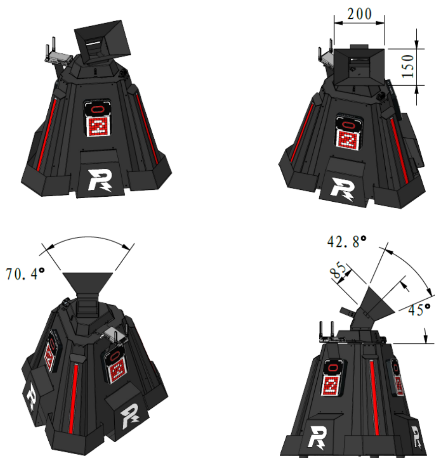
图 三-8 基地接收区示意图
