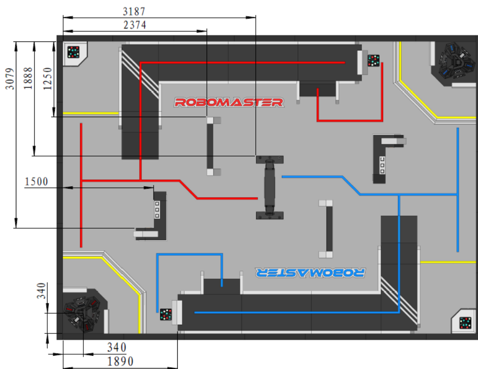
图 二-5 战场模块定位尺寸图
