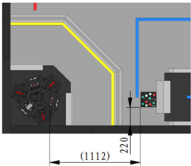
图 二-20 空中机器人识别卡
