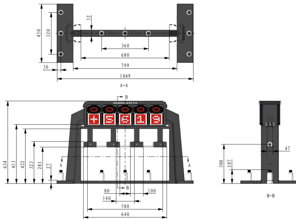
图 二-24 资源岛尺寸图
