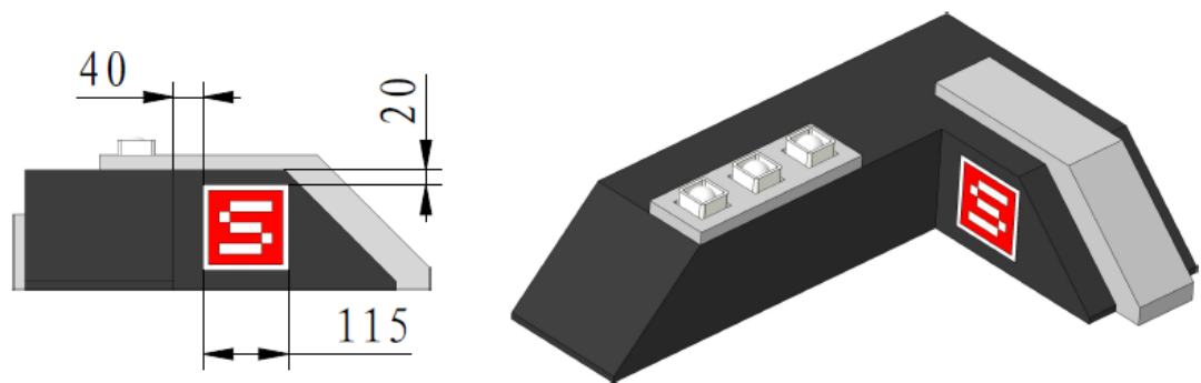
图 二-21 防御标签示意图
